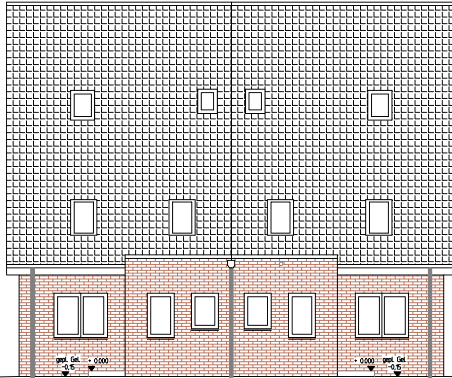
NORD-OST ANSICHT
