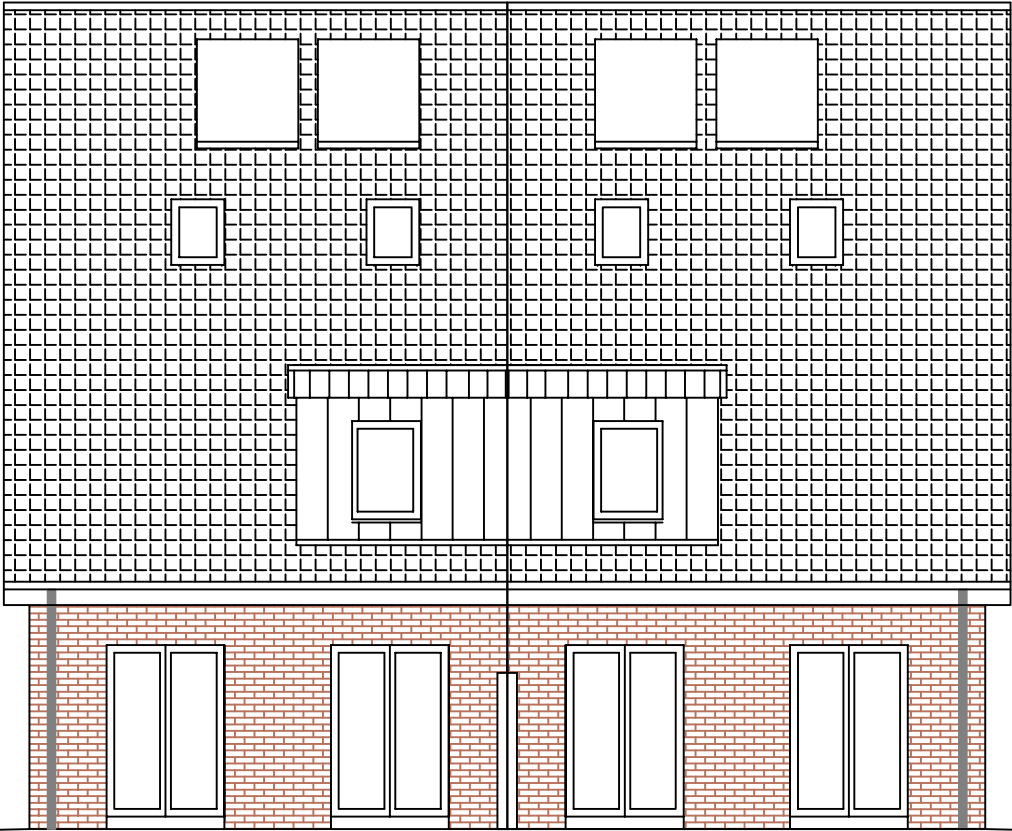
SÜD-WEST ANSICHT
