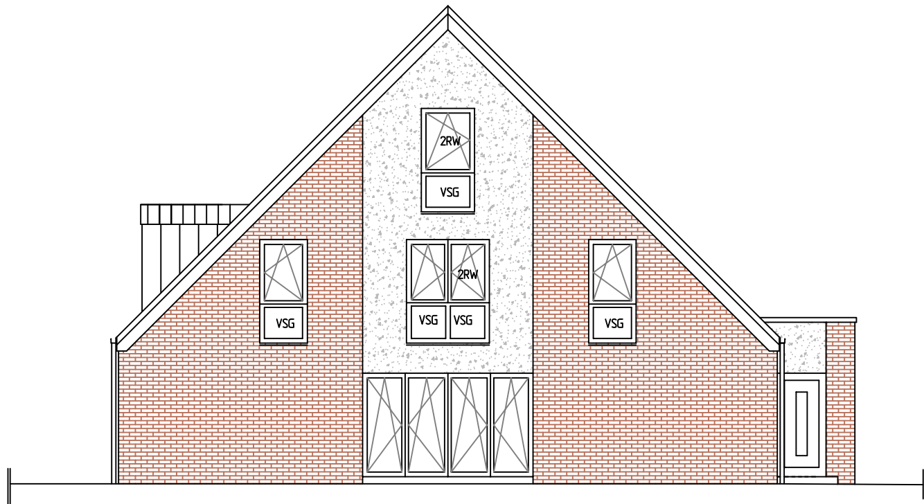
Giebelseite
