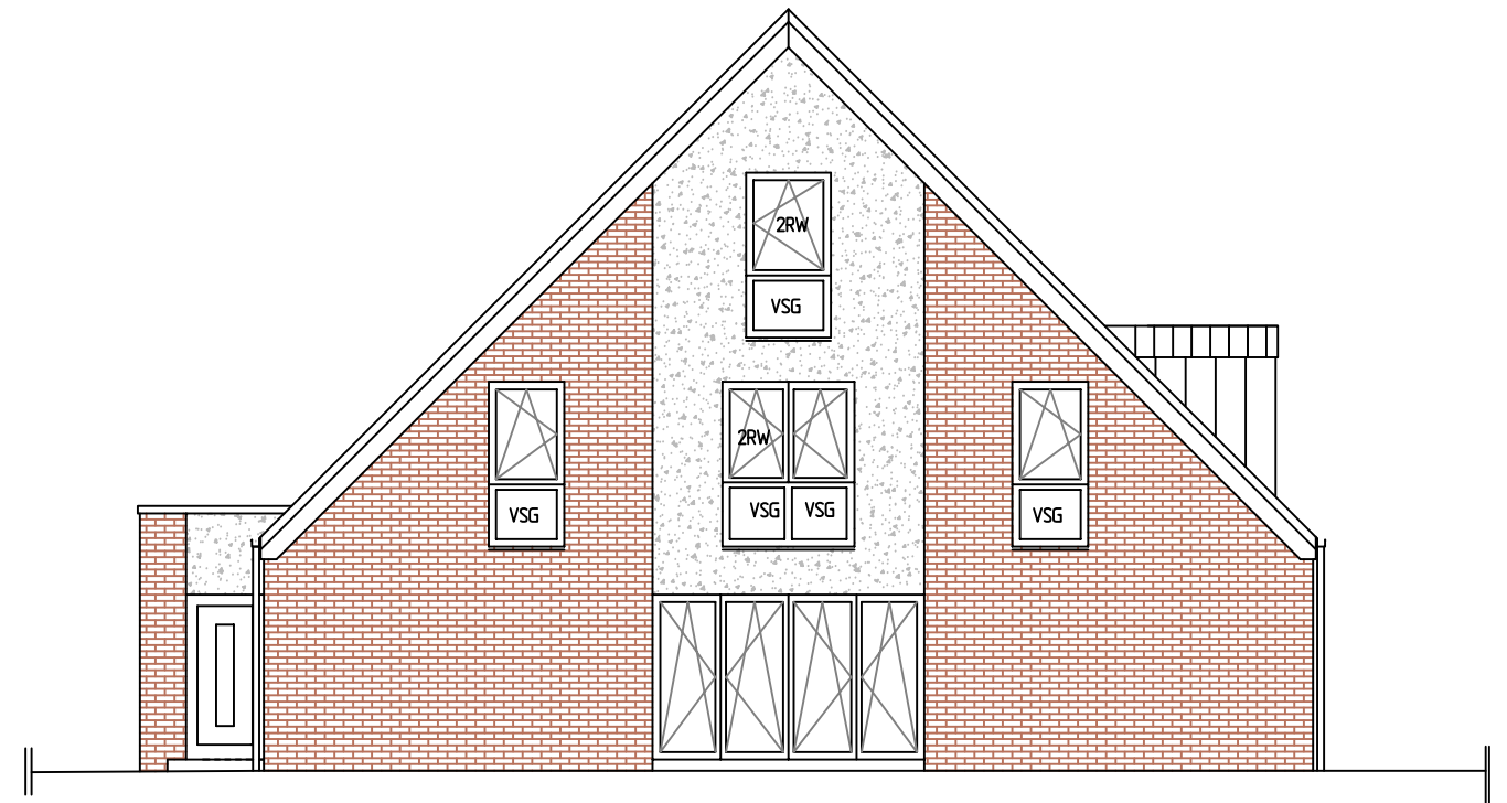
Giebelseite rechts
